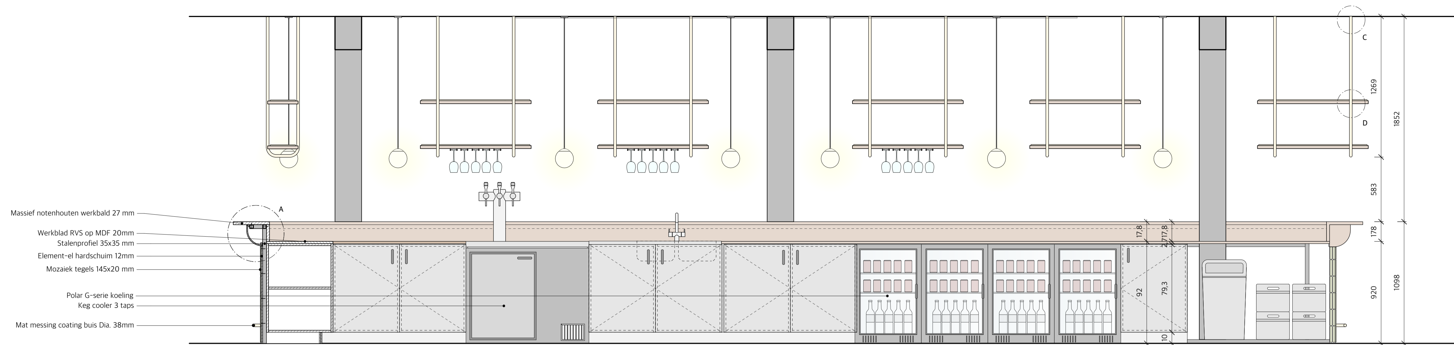
Achteraanzicht bar - 1/20
