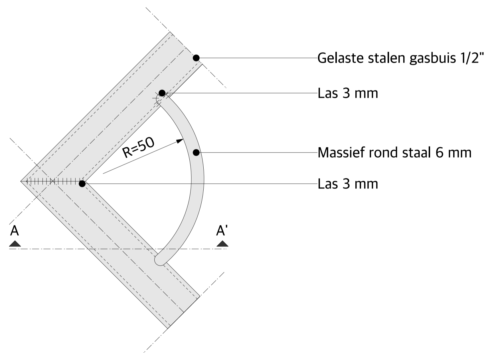
Bovenaanzicht
