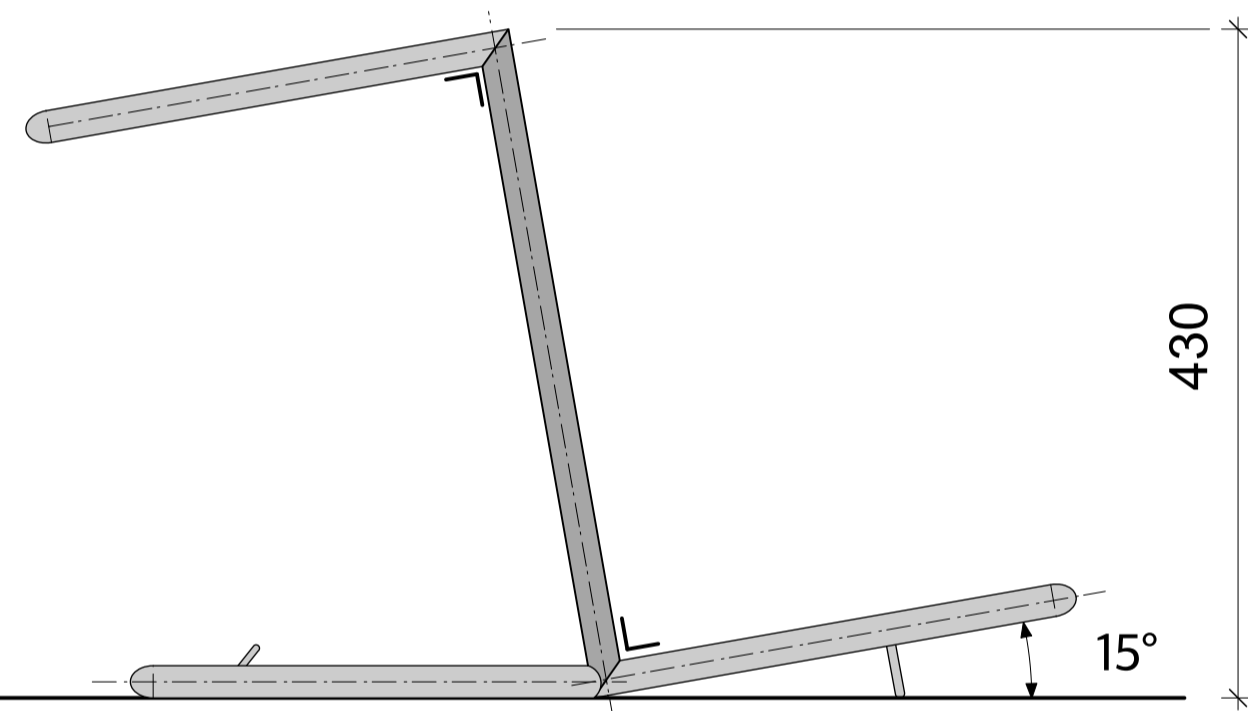
Zijaanzicht
