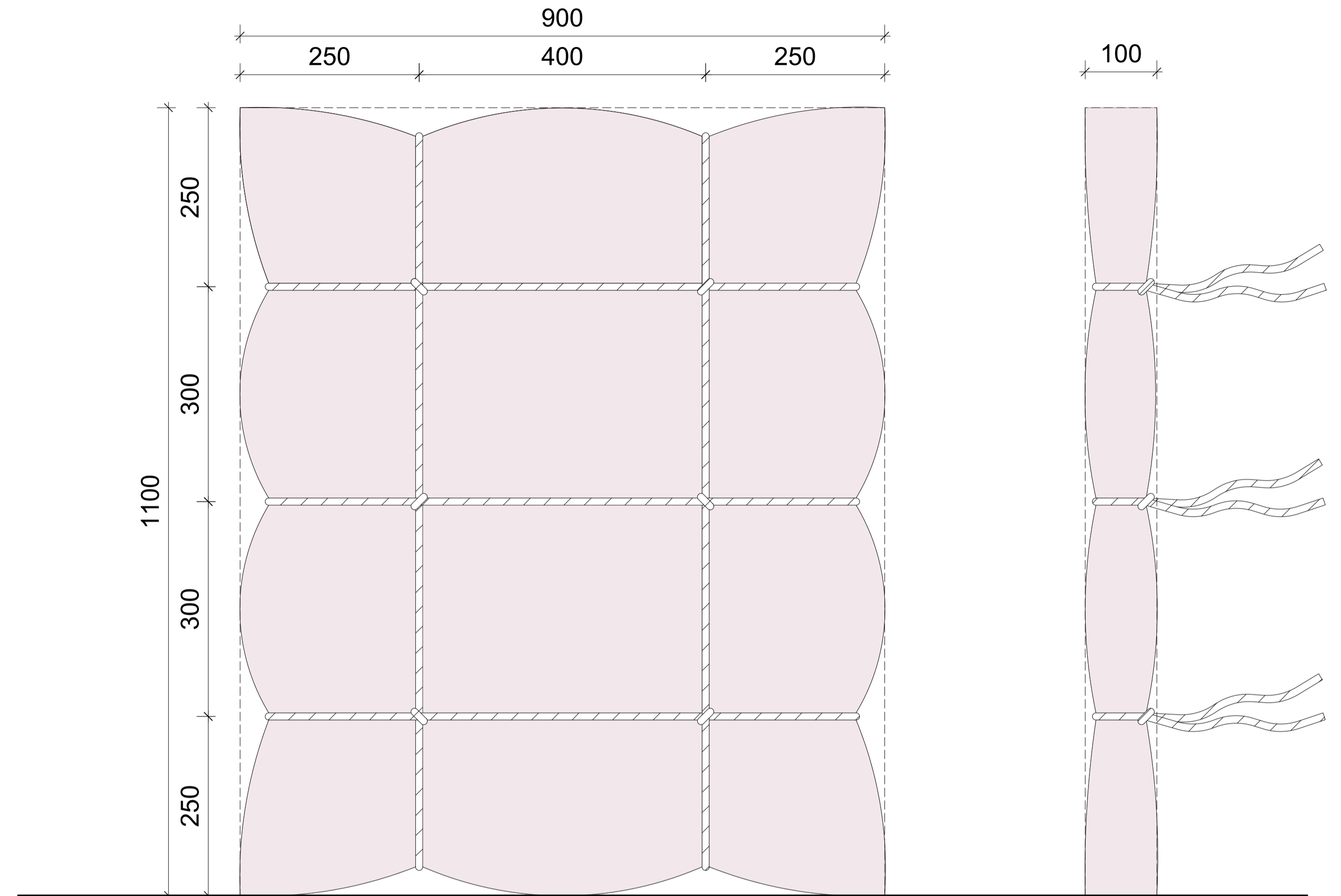
Vooraanzicht
