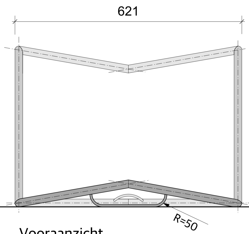
Vooraanzicht
